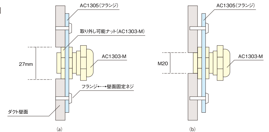
AC1303-M AC1305 組み合わせ図
