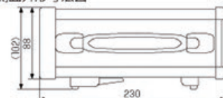
側面外形寸法図
