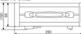
側面外形寸法図
