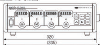
正面外形寸法図
