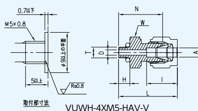
取付部寸法 VUWH-4XM5-HAV-V
