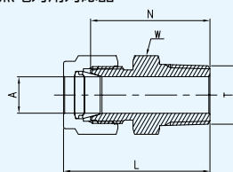
熱電対用対応品
