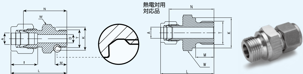
チューブ (インチサイズ) と ISO 平行おねじ
