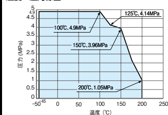
温度・圧力線図
