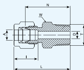
チューブ (ミリサイズ) とISOテーパーおねじ
