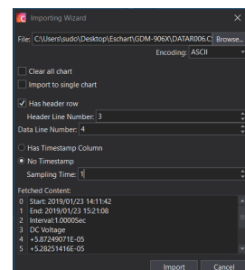
あらゆるCSV構造に対応
