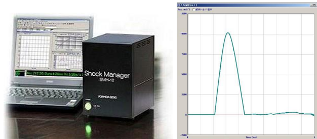
衝撃パルス例：1000G
